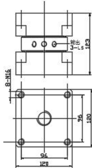
外形尺寸图
