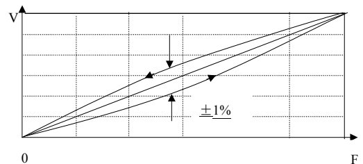
典型静态误差曲线 ( 三次取平均值 )
